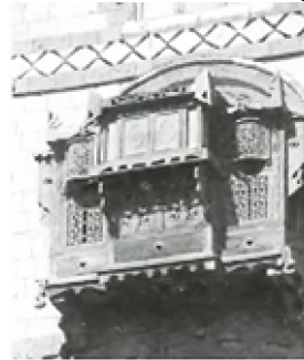
(شكل ١٩) الشاقوص للتهوية (شكل ٢٠) المشربية للتهوية
